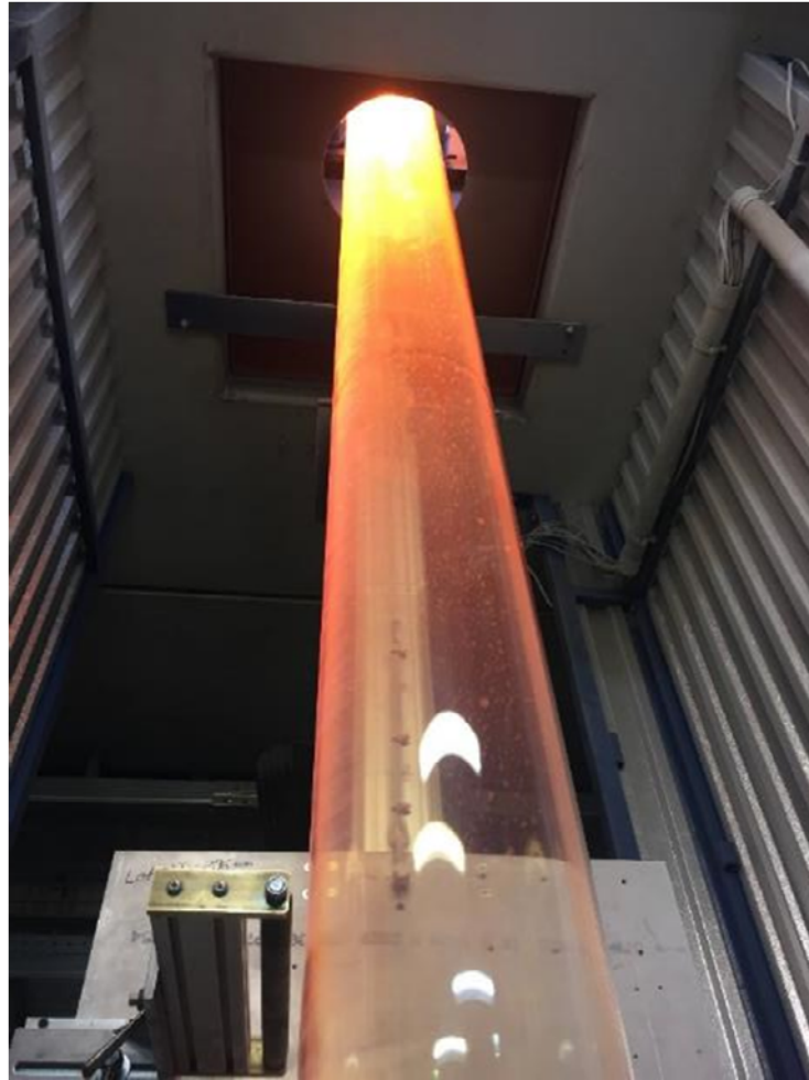
Glaszug für ein Rohr mit einem Durchmesser von 300 mm
