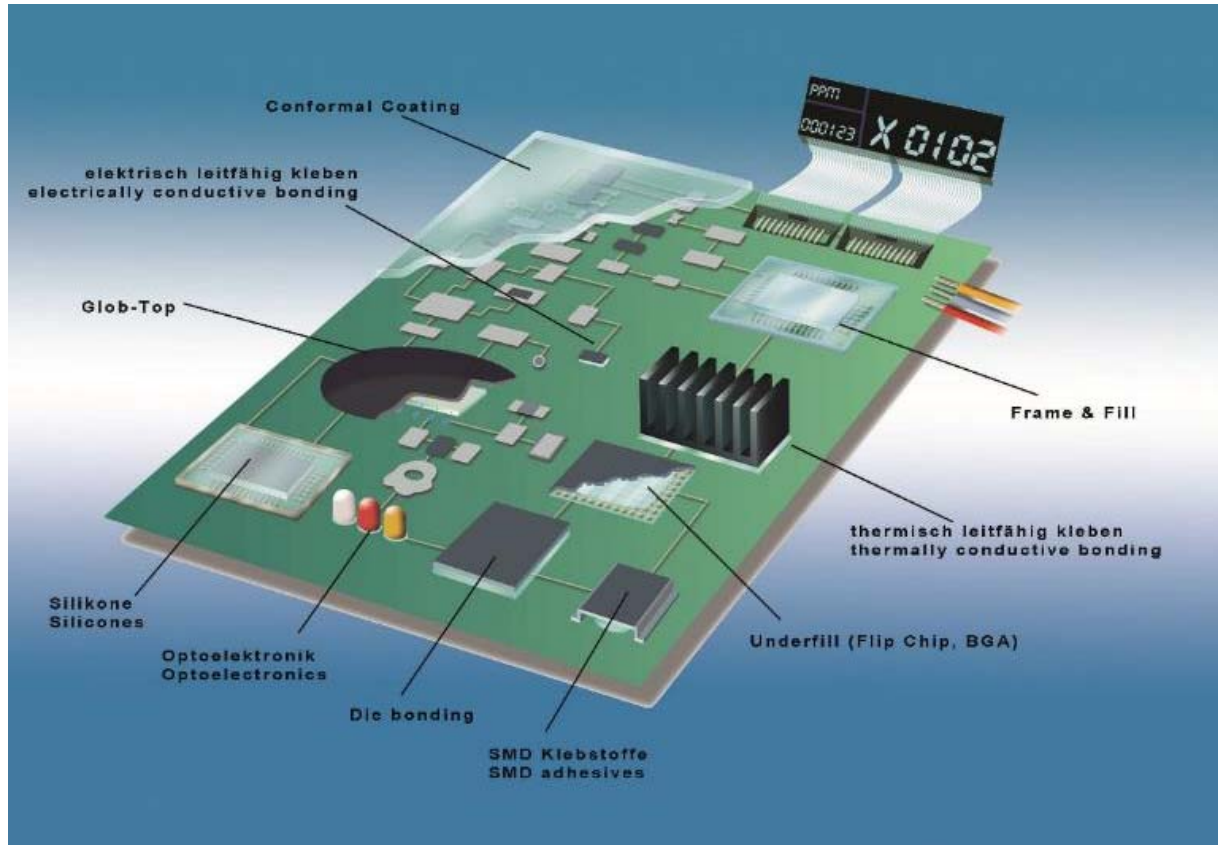
Mögliche Klebstoff-Anwendungen auf einer Leiterplatte
