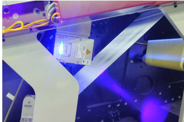
↑ PrintConcept LED auf einer Flexomaschine
