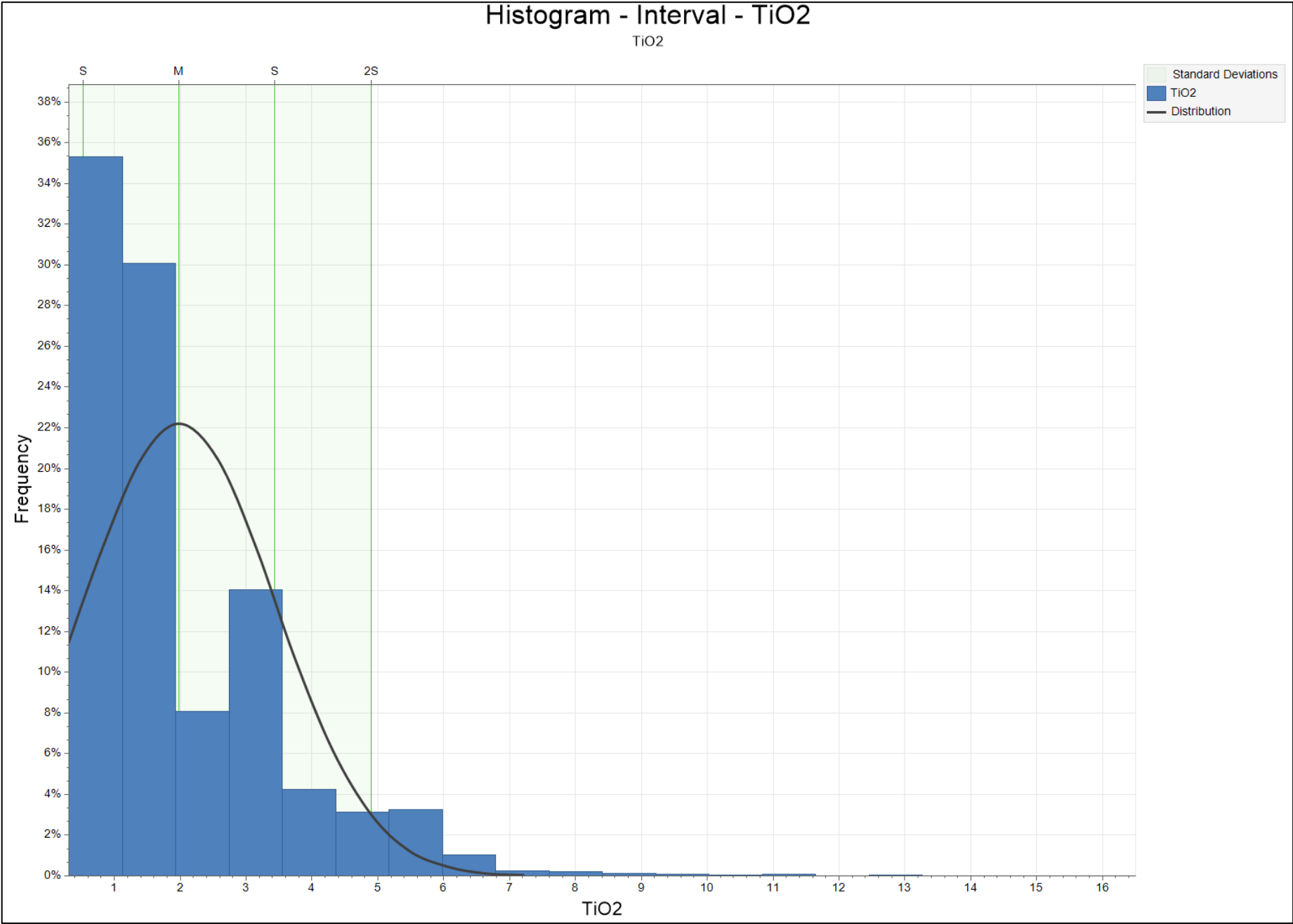
Figure 4.4 – TiO 2 Histogram
